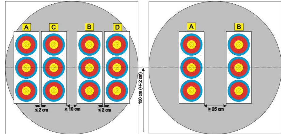
Placement de 4 tri spots
