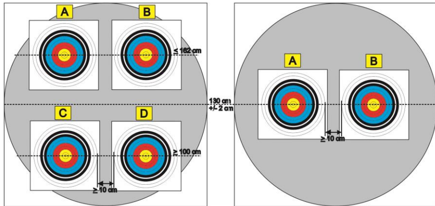
Plaatsing van 4 blaoenen 40 cm
