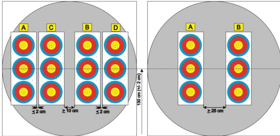
Plaatsing van 4 tri spots
